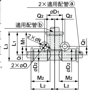
釋放套尺寸
