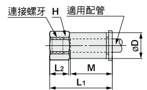
釋放套尺寸
