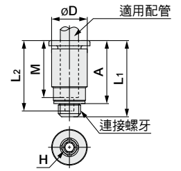
釋放套尺寸
