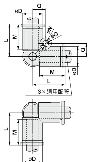
釋放套尺寸
