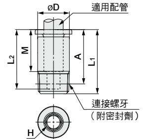
釋放套尺寸
