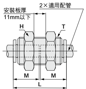
釋放套尺寸
