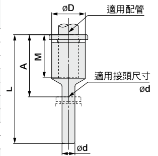
釋放套尺寸
