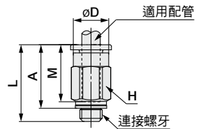
釋放套尺寸
