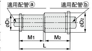
釋放套尺寸
