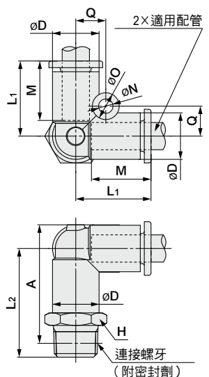
釋放套尺寸
