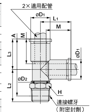
釋放套尺寸
