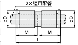
釋放套尺寸
