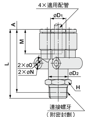
釋放套尺寸
