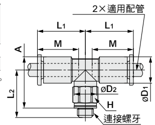
釋放套尺寸
